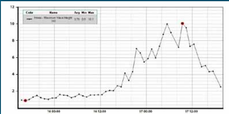
Met / Ocean: Maximum Wave Height (m)
